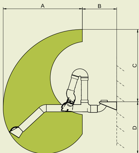
Seitansicht
